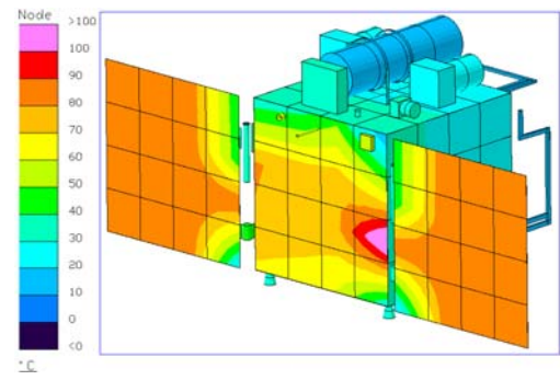
ب- طراحی شماره ۵، ۱/۰۲ متر لوله حرارتی
