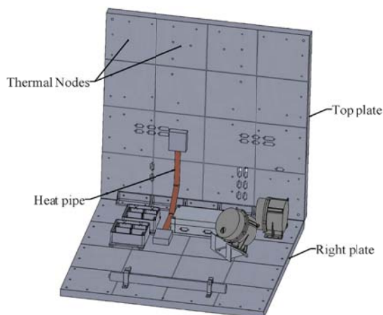
شکل ۴- شبکه‌بندی صفحات ماهواره به گره‌های حرارتی و نحوه اتصال لوله‌های حرارتی به این صفحات
