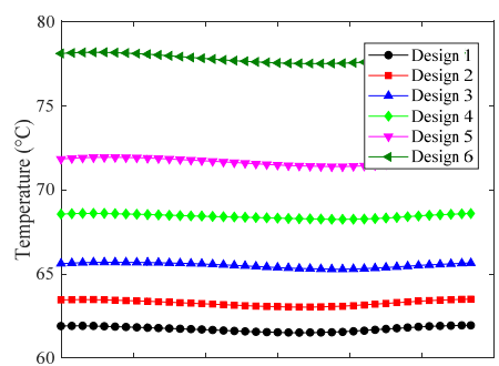
شکل ۱۳- دمای آرایه خورشیدی صفحه راست در \beta = 90^\circ
