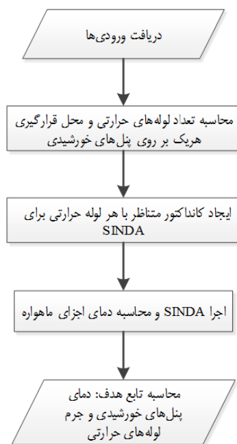
شکل ۳- فلوچارت محاسبه تابع هدف بهینه‌سازی
