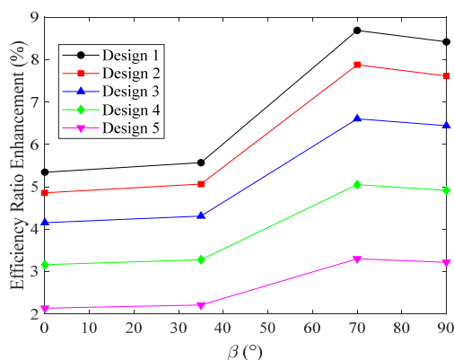
شکل ۲۶- افزایش نسبت بازده ( (\bar{\eta} - \bar{\eta}_{NHP}) / \bar{\eta}_{NHP} \times 100 ) سلول‌های خورشیدی صفحه‌ای راست در زوایای مختلف \beta
