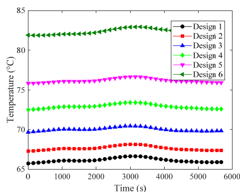
شکل ۱۴- دمای آرایه خورشیدی صفحه راست در \beta = 70^\circ
