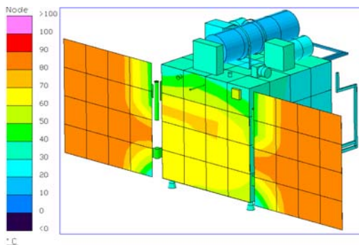
و- طراحی شماره ۱، ۵/۶۱ متر لوله حرارتی
