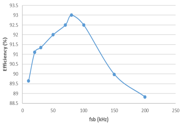
شکل ۱۱ - نمودار بازده مبدل نسبت به فرکانس کلیدزنی.
