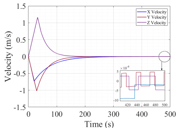
شکل ۹- سرعت فضاپیما تعقیب کننده
