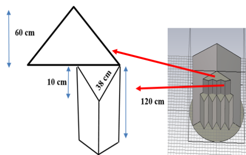
شکل ۸- ابعاد طبقه‌ی بالایی رفلکتور طرح دندان‌اره‌ای
