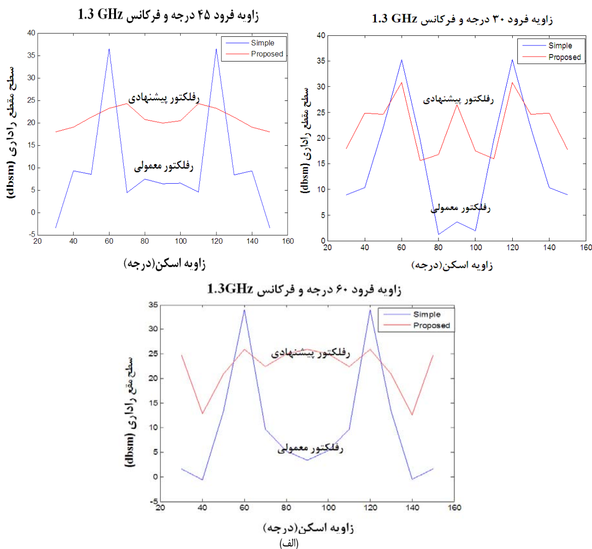
شکل ۹- مقایسه الگوی رفتاری رفلکتور معمولی و رفلکتور بهبود یافته در الف) فرکانس ۱/۳ GHz و زوایای فرود ۳۰، ۴۵ و ۶۰ درجه. ب) فرکانس ۵ GHz و زوایای فرود ۳۰، ۴۵ و ۶۰ درجه. ج) فرکانس ۱۰ GHz و زوایای فرود ۳۰، ۴۵ و ۶۰ درجه.
